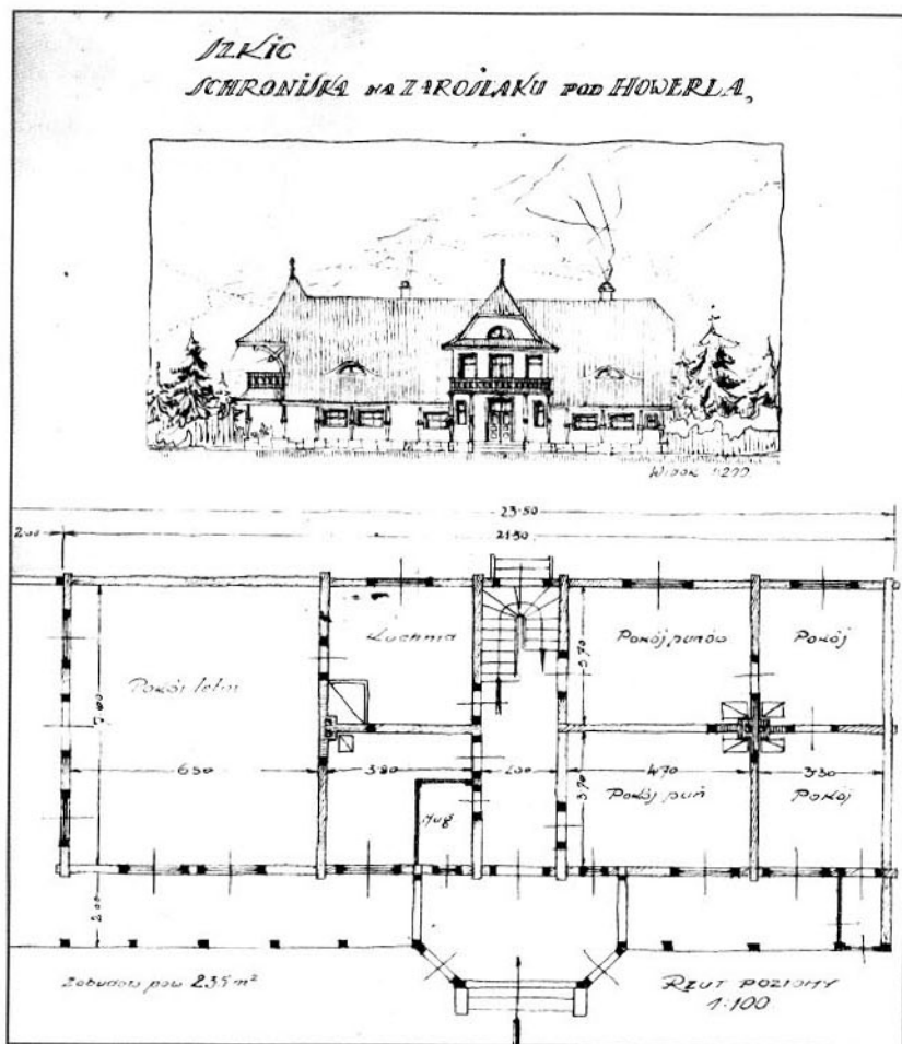
Проект схроніска Станіславівського відділу ПТТ на Заросляку, яке було збудоване в експлуатацію в 1927 р.
